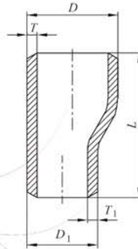
Zwężka mimośrodowa
